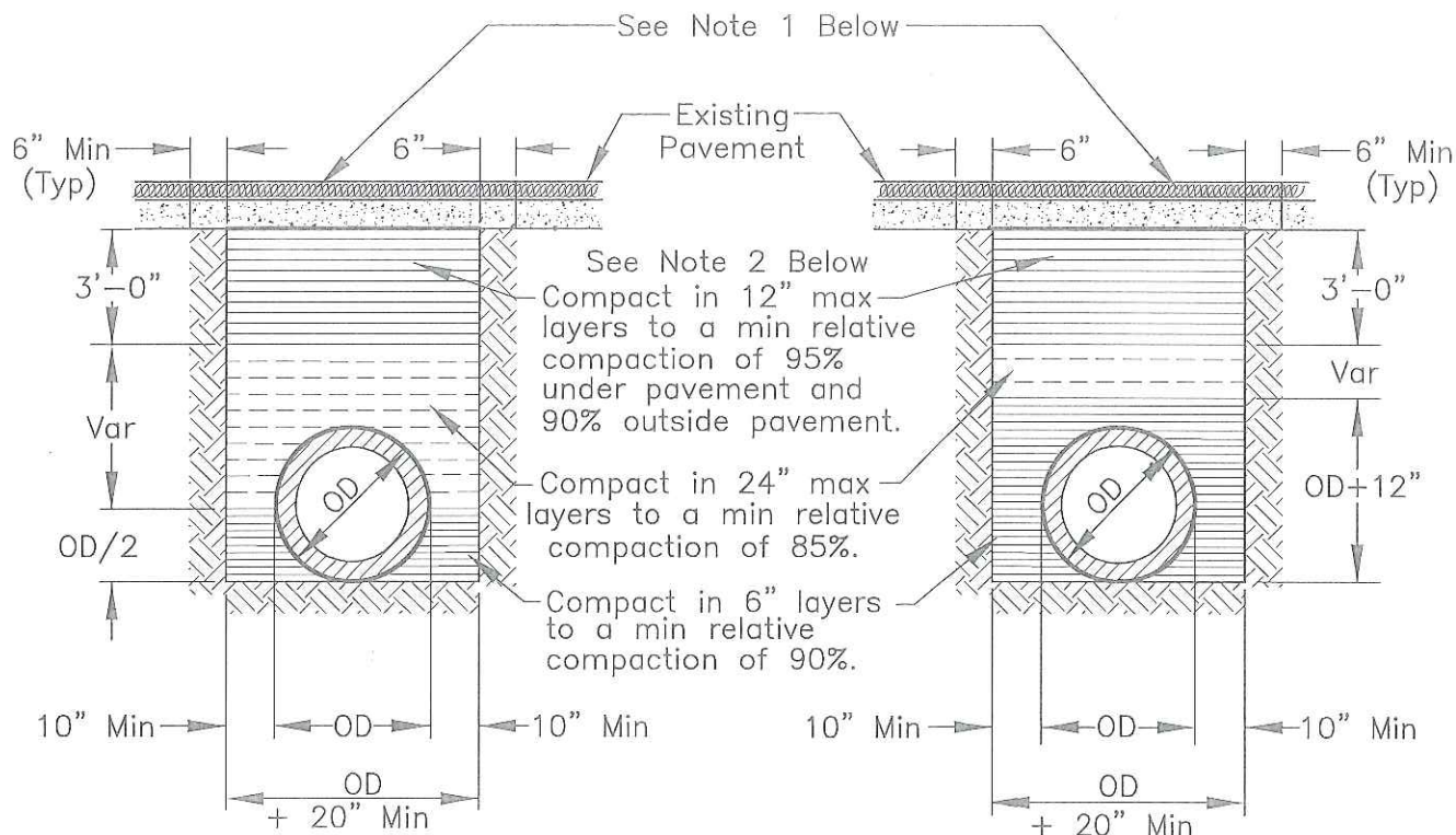
RIGID CONDUIT
